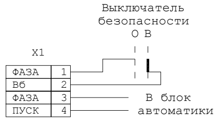
Схема подключения блока для работы с прибором «Мастер»
