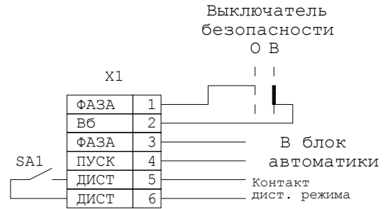
Схема подключения блока для работы с прибором «Текон»
