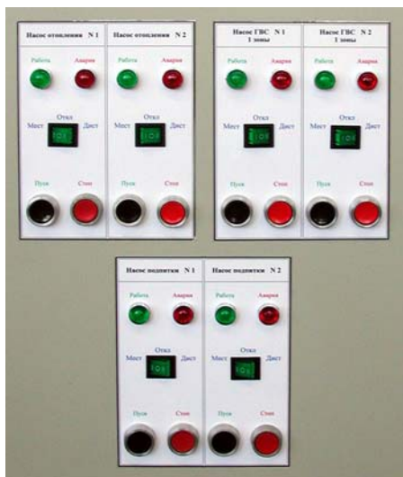
Лицевая панель щита ЩУ-1 с блоками управления шестью насосными агрегатами.
