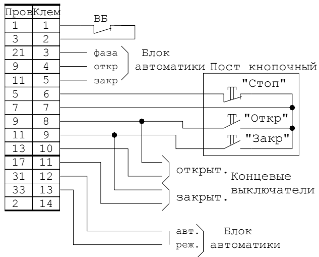
Схема подключения блока для работы с прибором «Мастер», «Текон». Для прибора «Мастер» клеммы 12 и 13 не используются.
